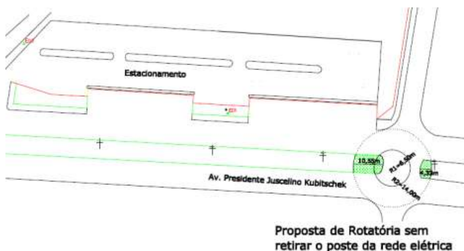
Figura 9 – Proposta de rotatória a ser implantada na Av. Pres. Juscelino Kubitschek.
